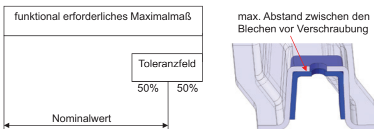
Bild 4.5 Nominalwert bei funktional erforderlichem Maximalmaß
