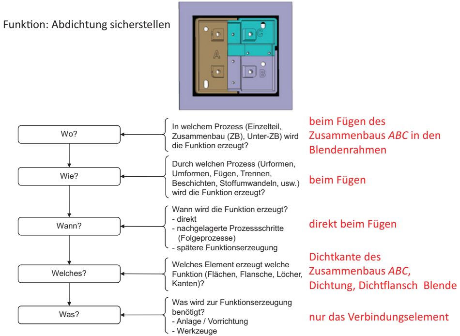
Bild 4.9 Anwendungsbeispiel zur Funktionsklärung
