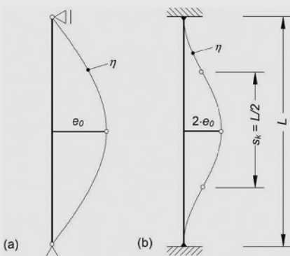
Bild K1. Ansatz der Imperfektionen bei einem gelenkig gelagerten Stab (a) und beidseitig eingespannten Stab (b) (nur qualitativer Vergleich)
