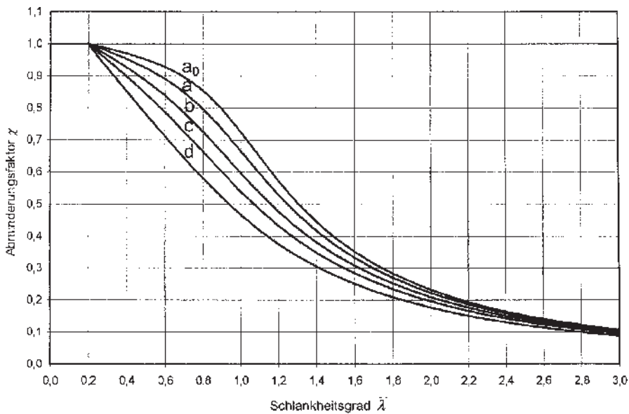
Bild 6.4. Knicklinien
